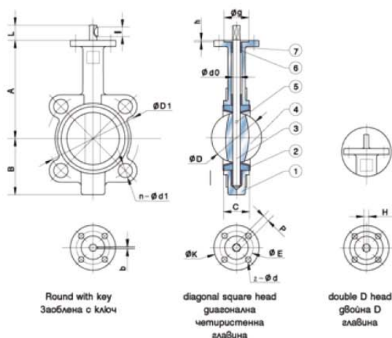
Wafer type / междифланцови тип
