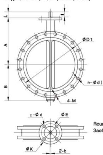
U Type / U Tip (с централен фланец)
